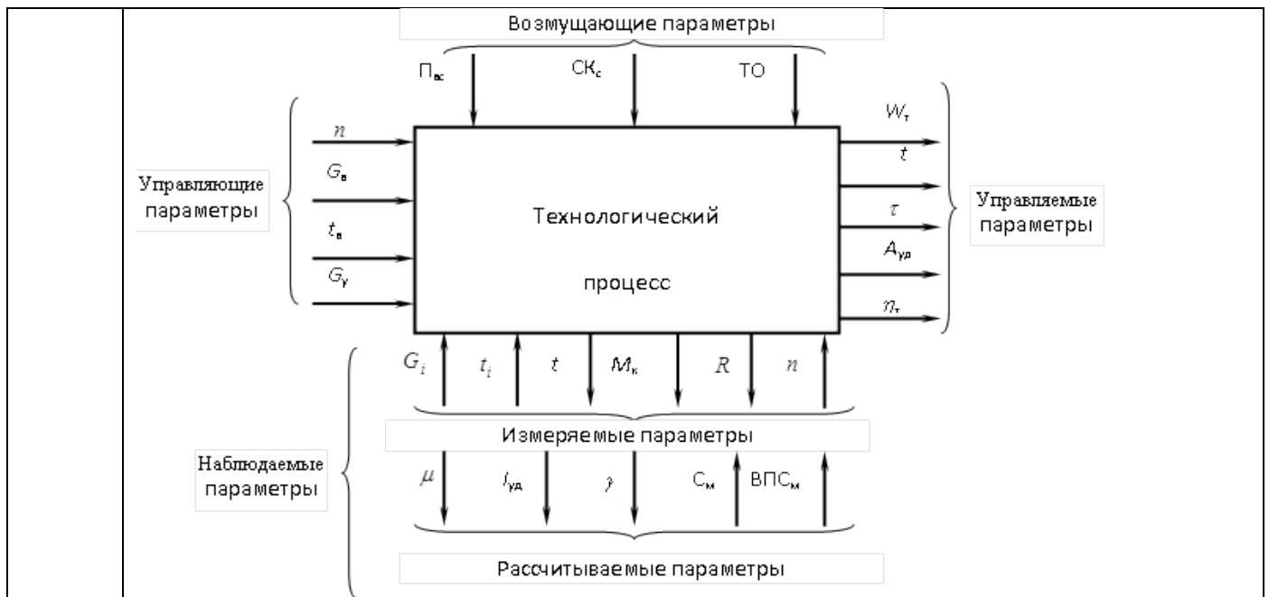
Рис. . Параметрическая схема процесса замеса теста
